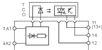
PIR6W-1PS-...-T, PIR6W-1PS-...-C, PIR6W-1PS-...-O
